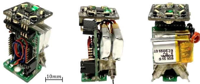
Fig. 12. mROBERTO millirobot.
